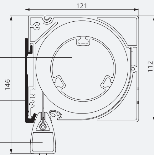
Geleidingsrail, hoekig
