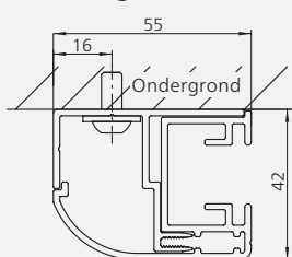
Geleidingsrail, rond
